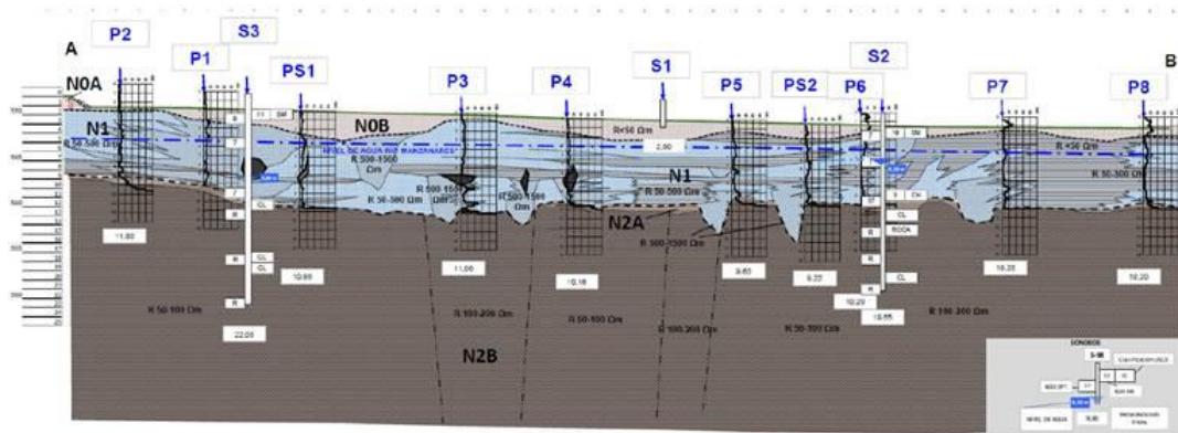
Imagen 3. Plano geotécnico sección transversal a ejecutar obras.
