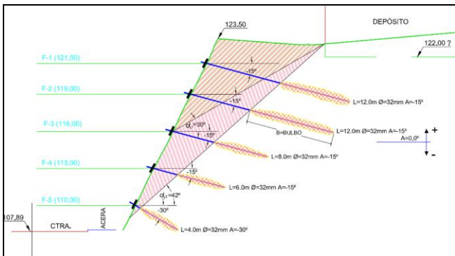
Sección tipo de unos de los taludes. Anclajes de barra Gewi de 32 mm + malla electrosoldada + hormigón proyectado.
