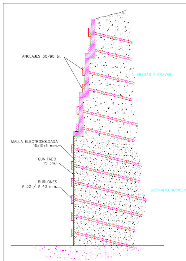
Sección típica del desmote con los elementos de estabilización: anclajes de 60 y 90 Tn – bulones en roca con barra tipo Gewi de 32 y 40 mm – mallazo electrosoldado y hormigón proyectado.
